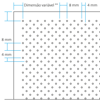
Perfuração Ø 1,5 mm Área perfurada ~ 5,5%
